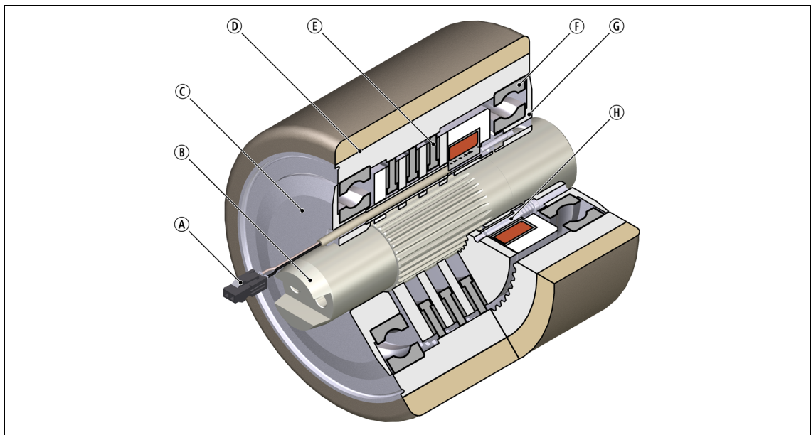
Abb. 1 Aufbau der Lamellen-Federkraftbremse INTORQ BFK453-08
