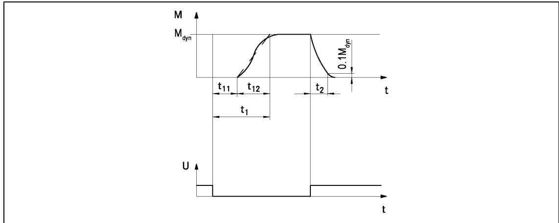
Abb. 3 Schaltzeiten der Federkraftbremsen
